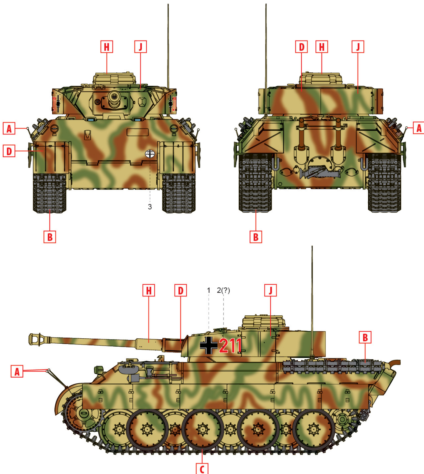
Bergepanther з баштою Pz.Kpfw.IV, 653-й важкий батальон винищувачів танків (Schwere Panzerjäger-Abteilung 653), 1944 рік Bergepanther with Pz.Kpfw.IV Turret, 653rd Heavy Panzerjäger Battalion (Schwere Panzerjäger-Abteilung 653), 1944
