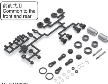
No.FAW302 FZアルミダンパーセット (FZ02/O2L/D2) FZ Aluminum Shock Set (FZ02/O2L/D2)
