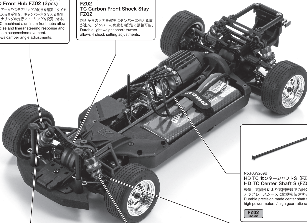
No.FAW205B HDフロントハブ FZ02 (2個入) HD Front Hub FZ02 (2pcs)
