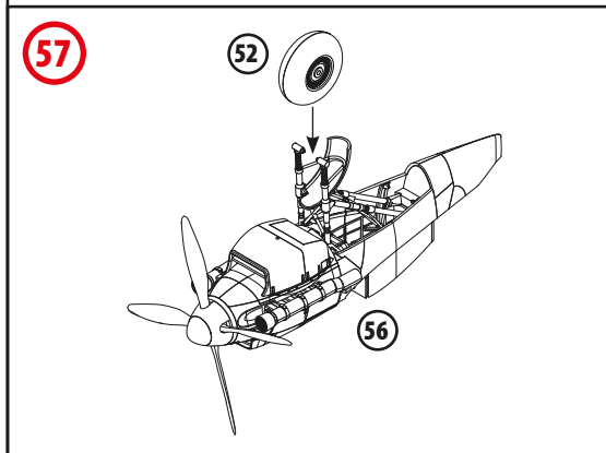
ЛЕВАЯ МОТОГОНДОЛА LEFT ENGINE NACELLE
