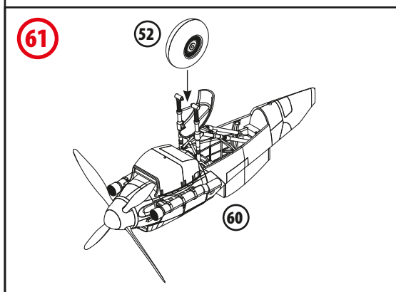
ПРАВАЯ МОТОГОНДОЛА RIGHT ENGINE NACELLE
