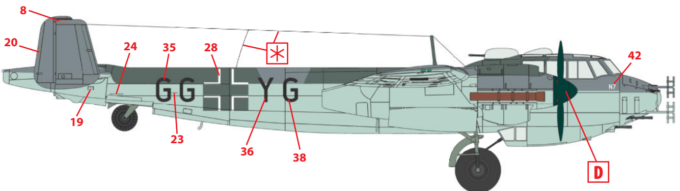
Другой вариант окраски Another painting variant
