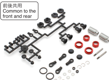
No.FAW302 FZアルミダンパーセット (FZ02/O2L/D2) FZ Aluminum Shock Set (FZ02/O2L/D2)
