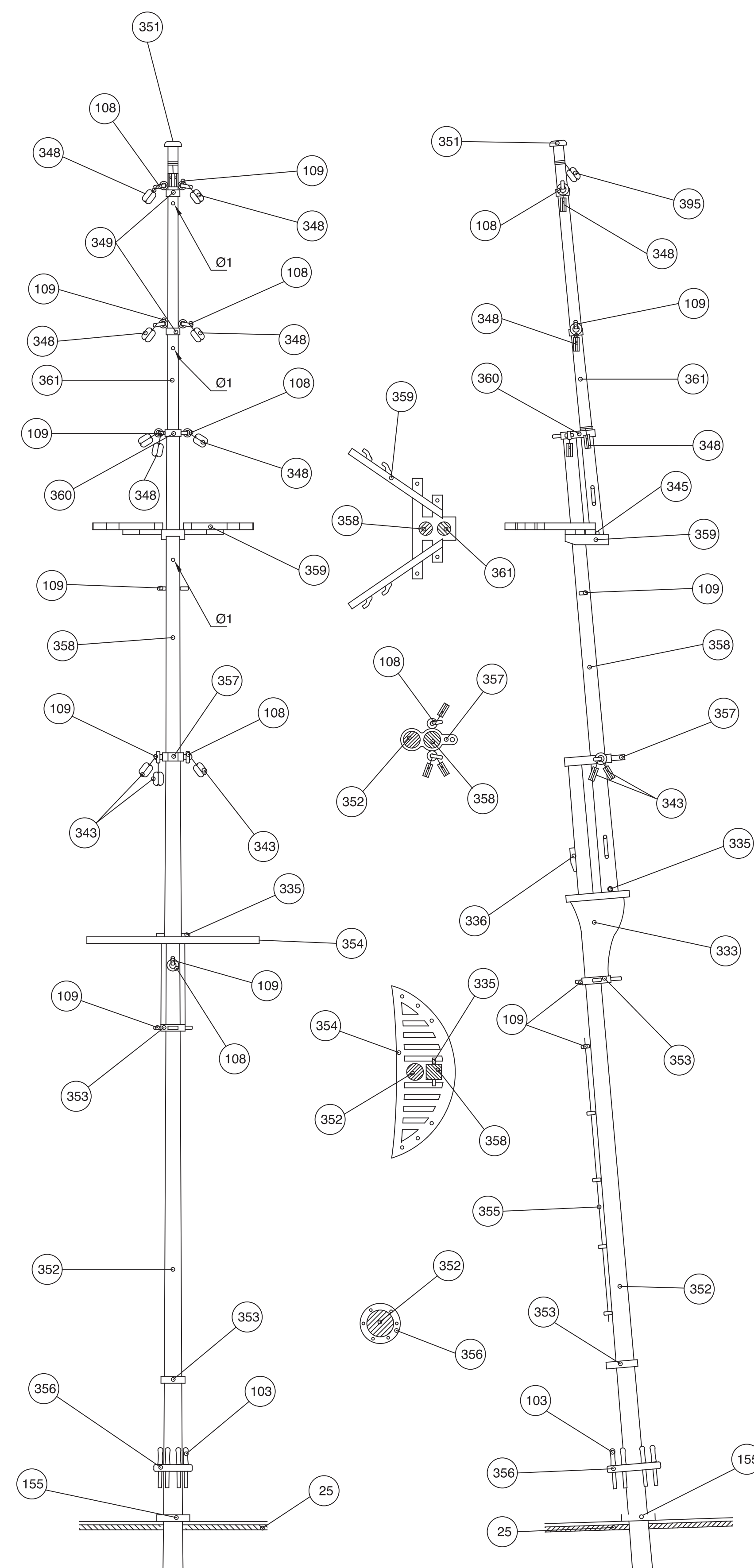
Palo mesana Mizzen mast Mât d'artimon Besanmast Albero di mezzana Mastro do mezena Bezaansmast
