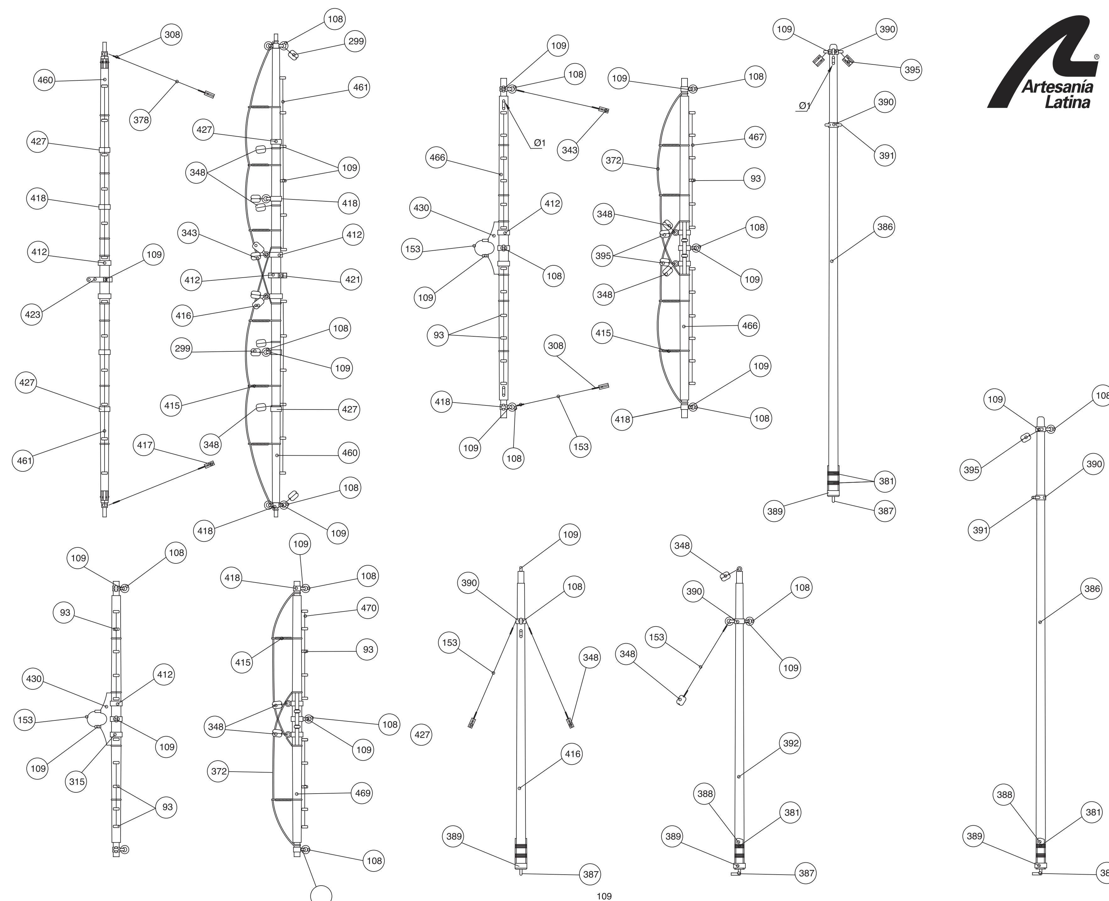
Bauprés Bowsprit Beaupré Bugsprit Bompresso Bergantim Boegsprit
