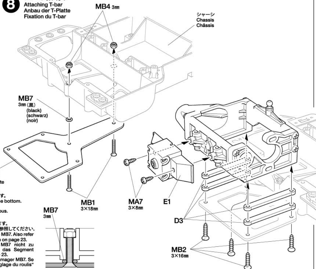
3×16mm皿タッピングビス Tapping screw Schneidschraube Vis taraudeuse
