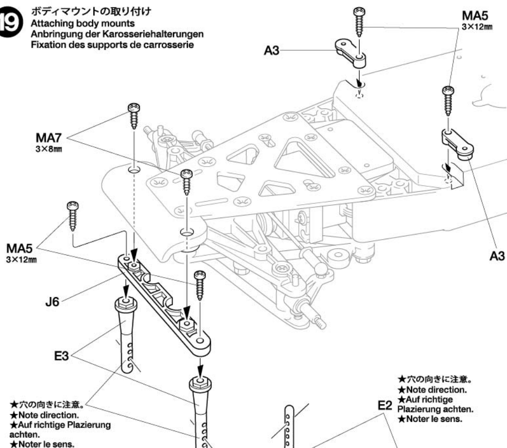
MA5 ×6 3×12mmタッピングビス Tapping screw Schneidschraube Vis taraudeuse
