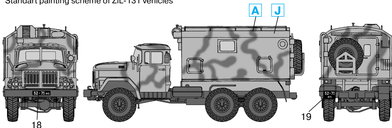
Камуфляжная окраска автомобилей «Зил-131» Camouflage painting scheme of ZiL-131 vehicles
