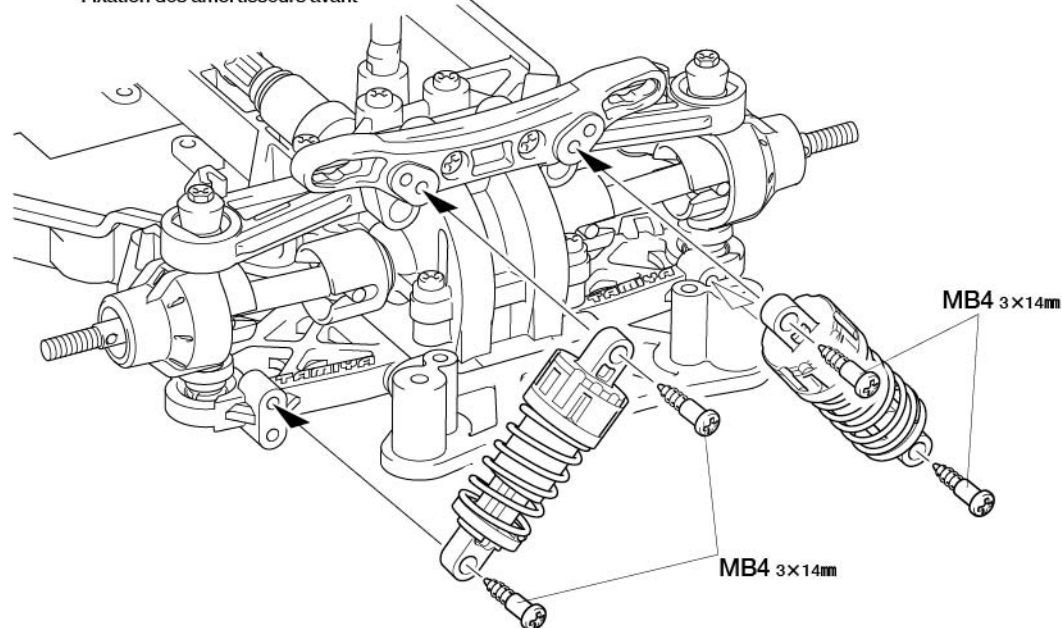
MB4 x4 3×14mm段付タッピングビス Step screw Paßschraube Vis décolléte
