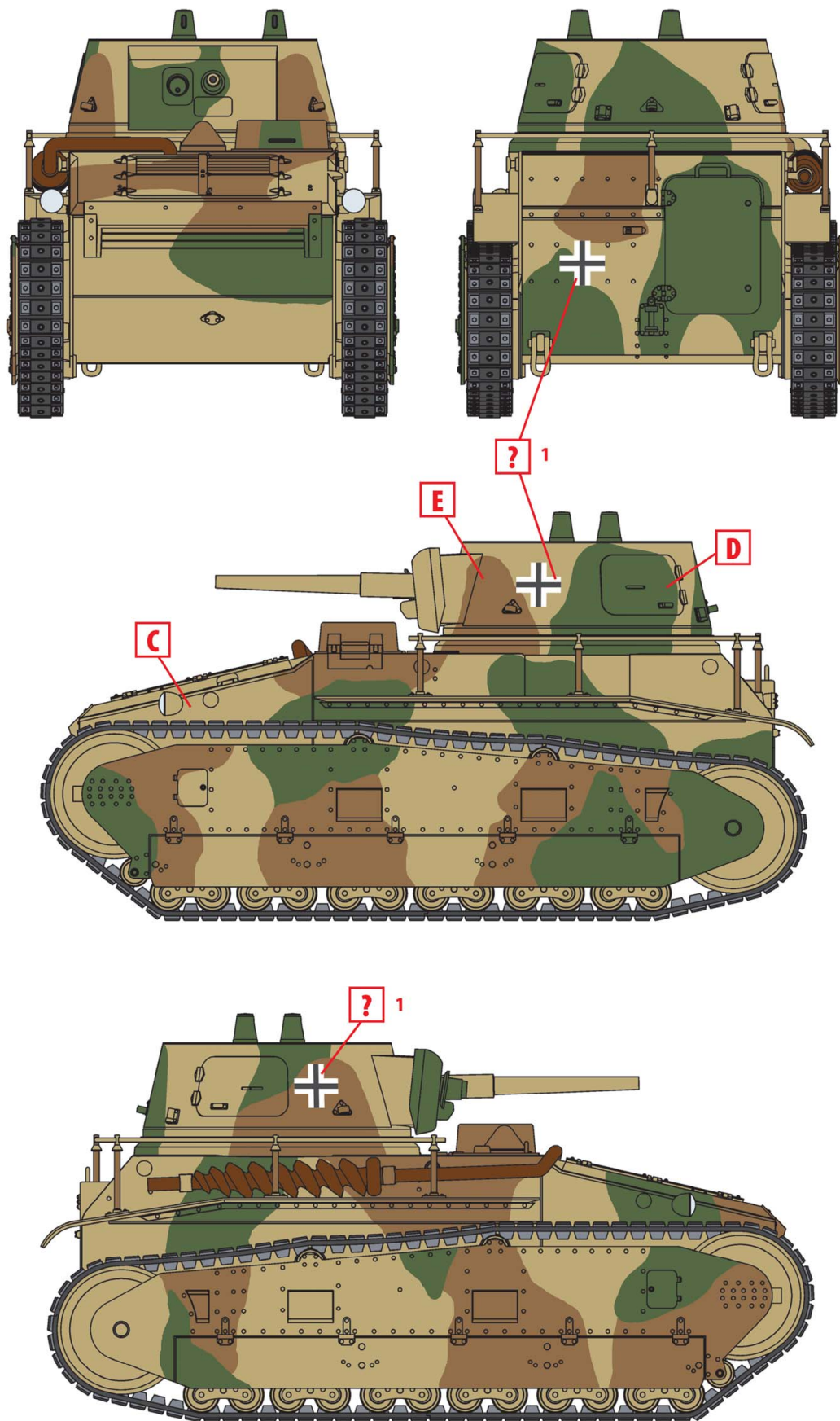
“Легкий трактор” Рейнметалл, Германия, 1930 г. Leichttractor Rheinmetall, Germany, 1930
