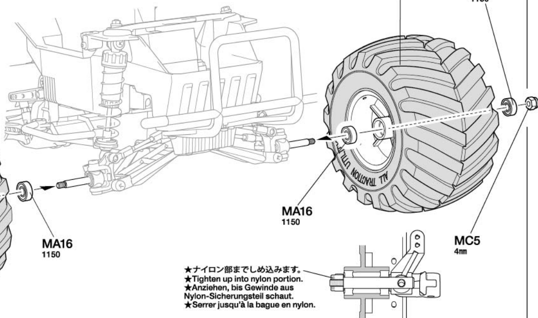
MA16 ×4 1150ベアリング Ball bearing Kugellager Roulement à billes
