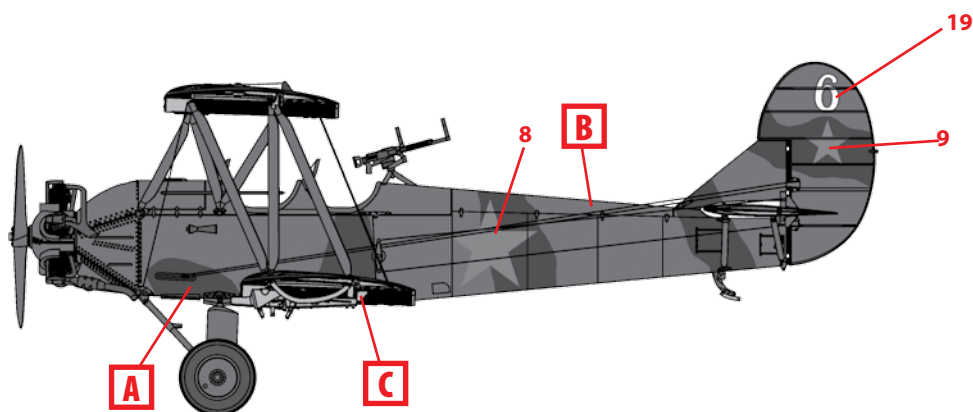
У-2ВС из 213-й НБАД, лето 1943 г.
