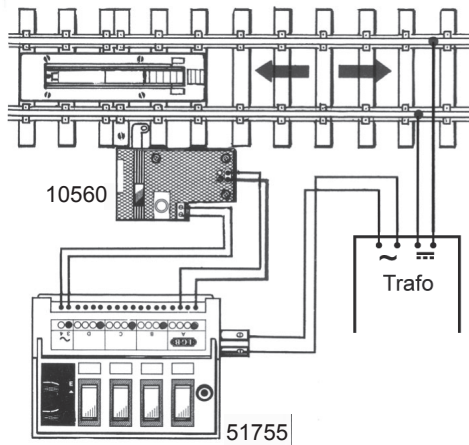
Bild 3 Elektrischer Anschluss des Entkupplungsgleises
