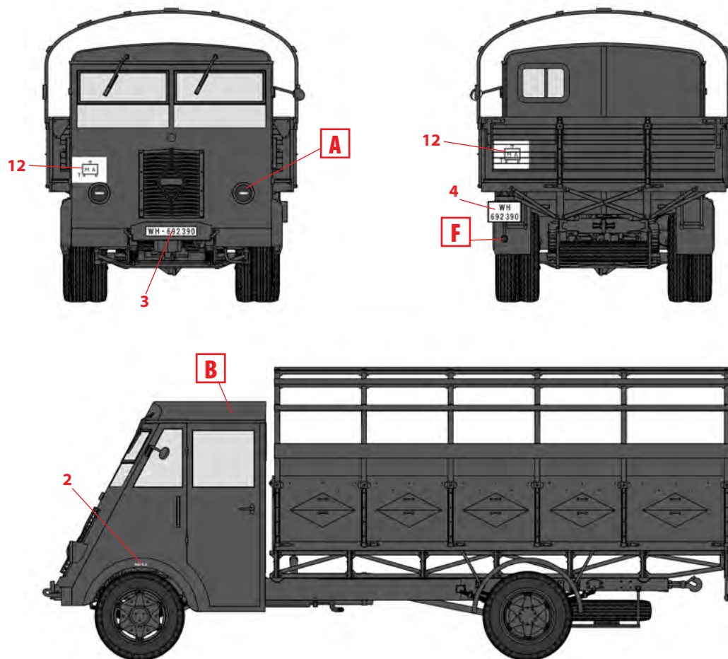
1. Lastkraftwagen 3,5 t AHN, Россия, зима 1941 г. Lastkraftwagen 3,5 t AHN, Russia, Winter 1941
