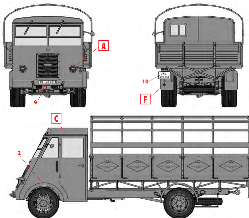
4. Lastkraftwagen 3,5 t AHN, Италия, 1943 г. Lastkraftwagen 3,5 t AHN, Italy, 1943
