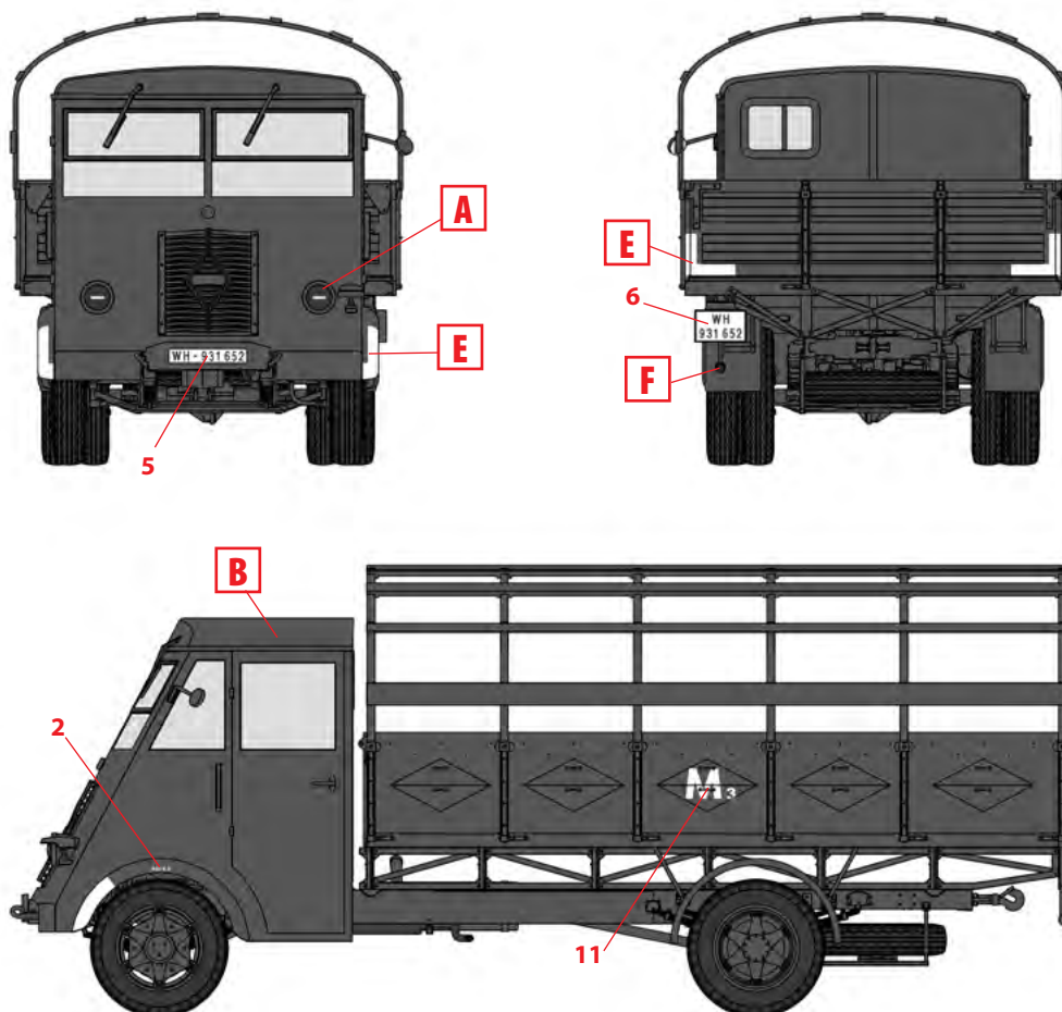
2. Lastkraftwagen 3,5 t AHN, Украина, лето 1942 г. Lastkraftwagen 3,5 t AHN, Ukraine, Summer 1942
