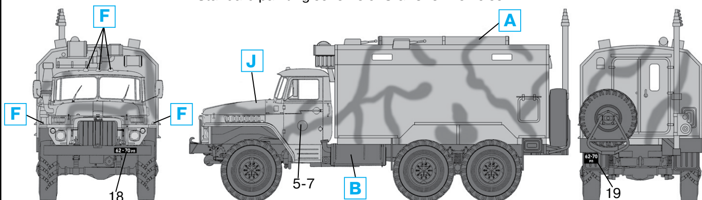
Камуфляжная окраска автомобилей «Урал-375А» Camouflage painting scheme of Ural-375A vehicles
