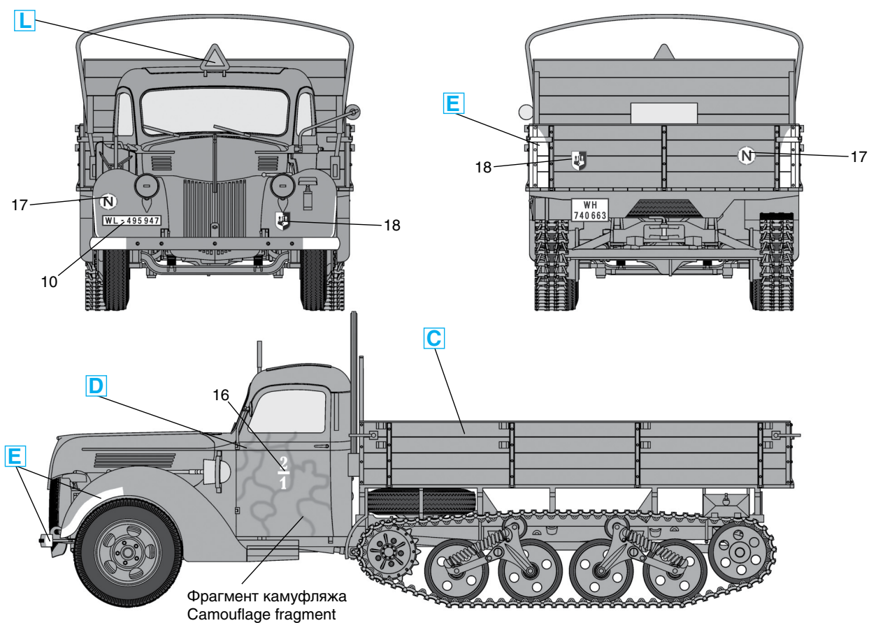
V3000S/SS M (Kfz.3b) Maultier, Италия, лето 1944 г. V3000S/SS M (Kfz.3b) Maultier, Italy, Summer 1944
