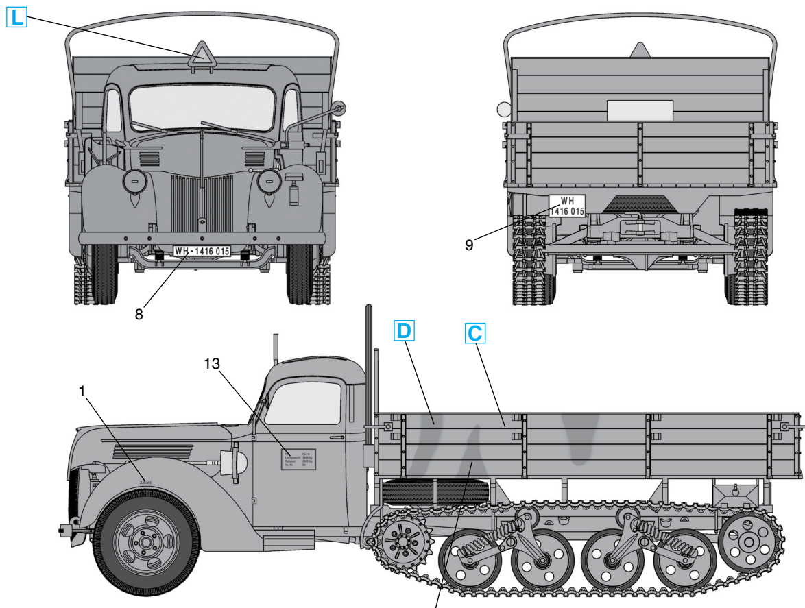
V3000S/SS M (Kfz.3b) Maultier, Польша, лето 1944 г. V3000S/SS M (Kfz.3b) Maultier, Poland, Summer 1944
