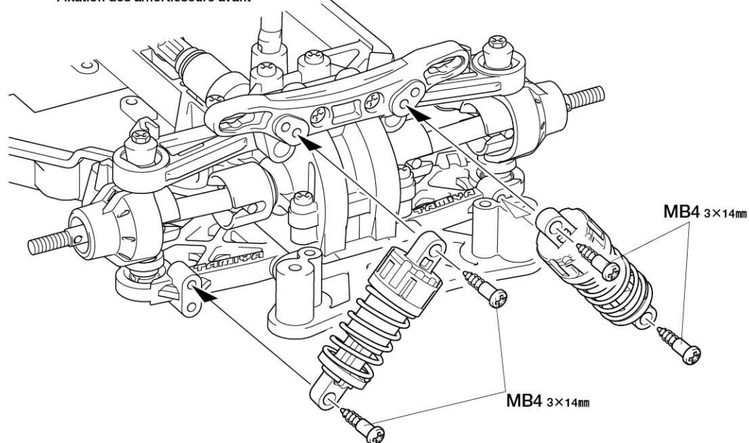
MB4 ×4 3×14mm 段付タッピングビス Step screw Paßschraube Vis décollétée
