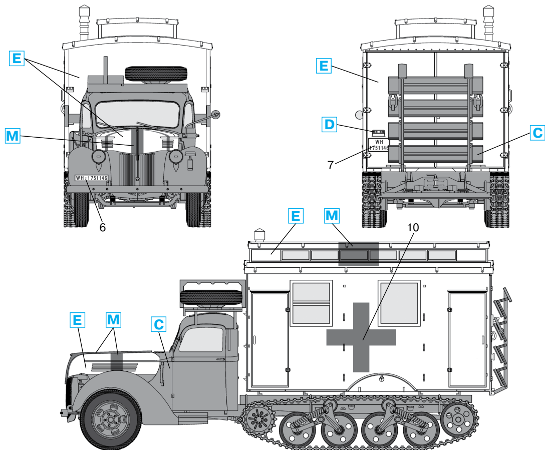
V3000S/SS M Maultier с будкой, Польша, осень 1944 г. V3000S/SS M Maultier with Shelter, Poland, Autumn 1944
