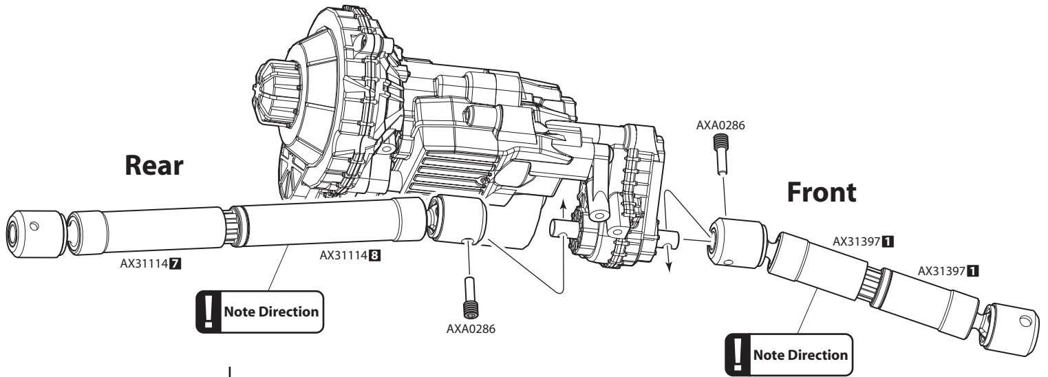
AXA0286 M4x2.5x13mm x2
