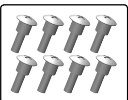
C-00250-026 Vis épaulées - Acier - 8 pcs
